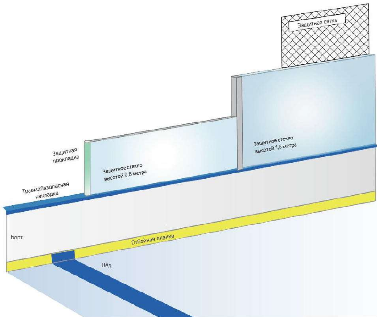
Рисунок 13. Борт, защитное стекло и защитная сетка
