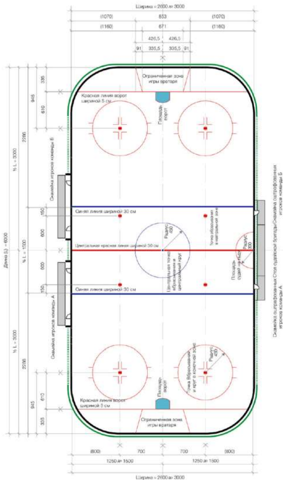
Рисунок 3. Размеры стандартной игровой площадки
